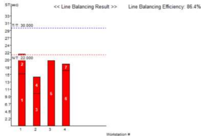
Gambar 6. Efisiensi Hasil Optimasi Takt Time
